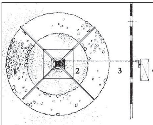
▲ Schematische plattegrond van een rosmolen, type geubel. Verklaring gebruikte nummers: 1: rosmolenpad; 2: geubel; 3: aandrijfjas; 4: aan te drijven apparaat/machine.
