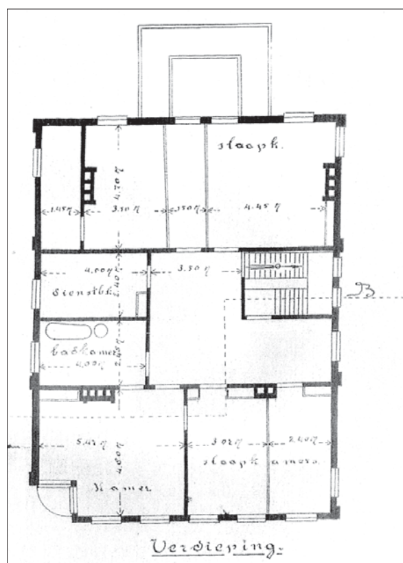
▲ De plattegronden van de begane grond en de eerste verdieping
