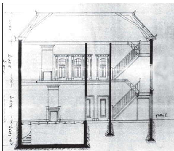
►▲ Bouwtekening van de achtergevel van de notariswoning met daarin de serre deuren van de voormalige woning (zie foto pagina 21)
