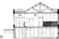
Doorsnede secretarie
