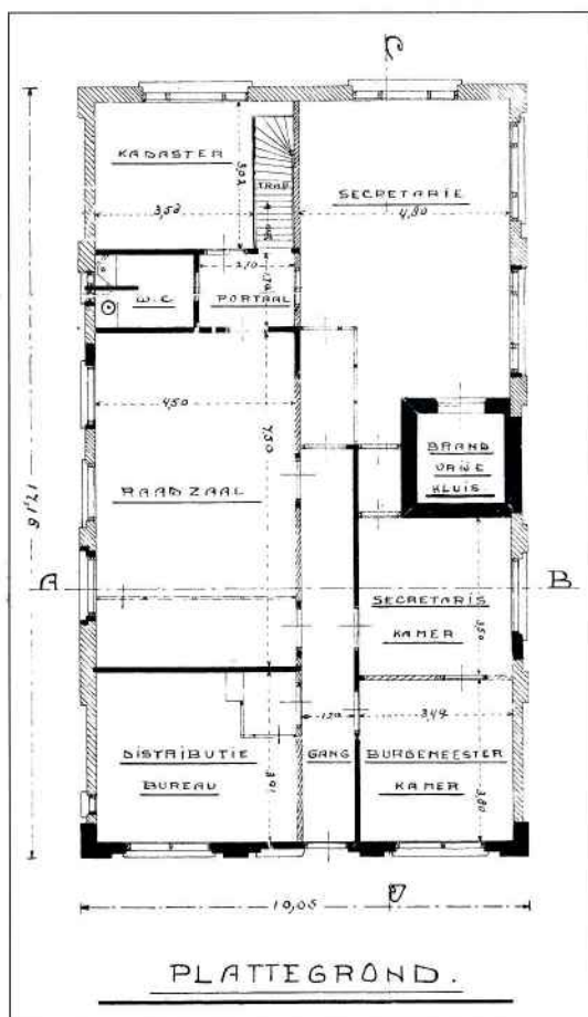
Plattegrond voor de verbouwing van het gemeentehuis aan de Schoolstraat (1917).
